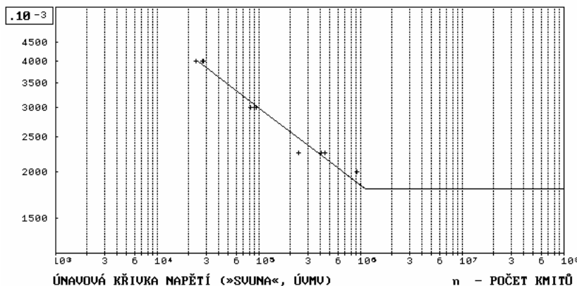
Obrázek 3 - Wöhlerova křivka úplného ramene přední nápravy ŠKODA Favorit, náhradní provedení
