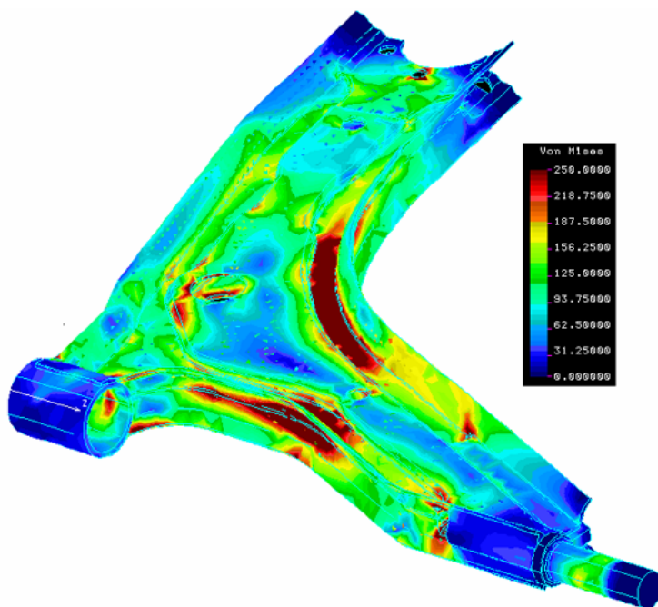
Obrázek 2 – MKP analýza ramene přední nápravy při zatížení popdélnou silou 4kN
